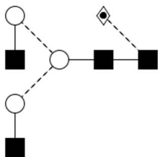
Oxford Notation
