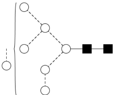
Oxford Notation
