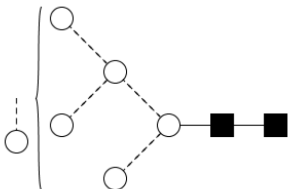
Oxford Notation
