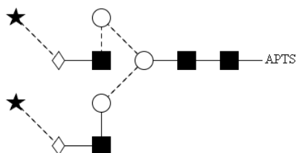
Oxford Notation
