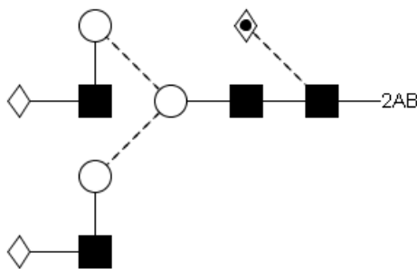
Oxford Notation
